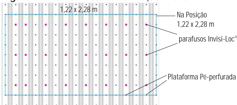
Figura A Invisi-Loc ® Sistema de Fixação Inferior
