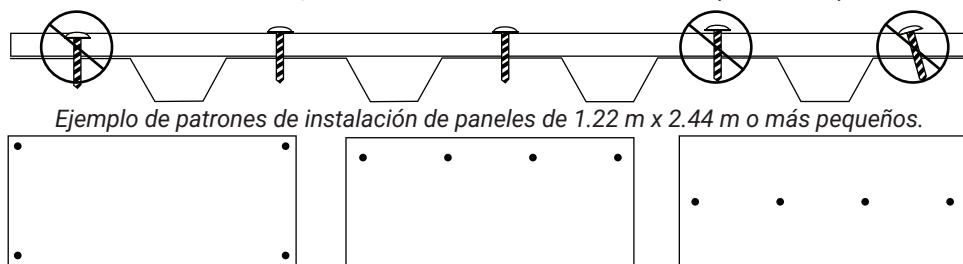
Figura F - Instalación de tornillos ESD
